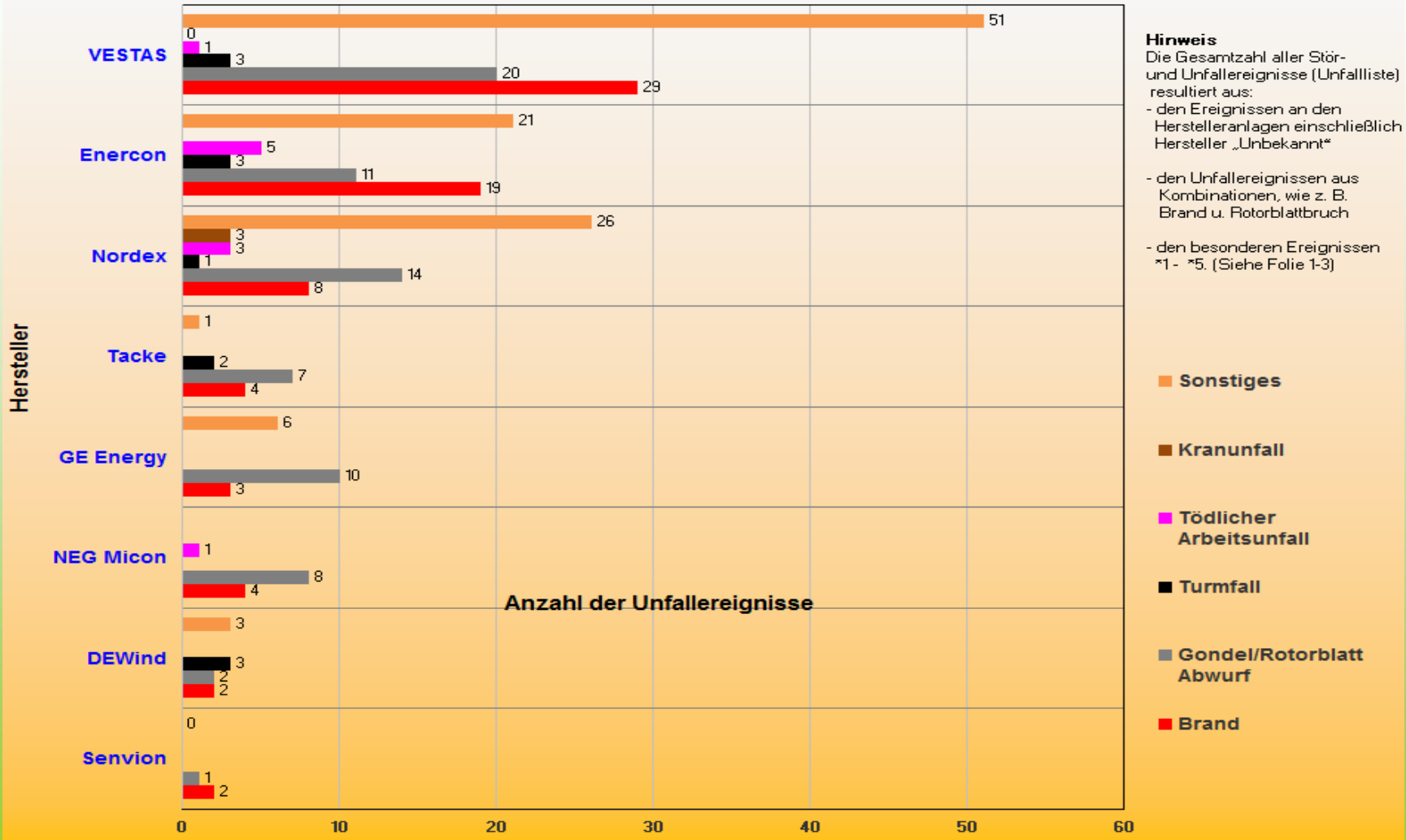
Stör- u. Unfallereignisse an Windkraftanlagen nach Unfallhäufigkeit (Erfassungszeitraum 2000 - 12/2025)
